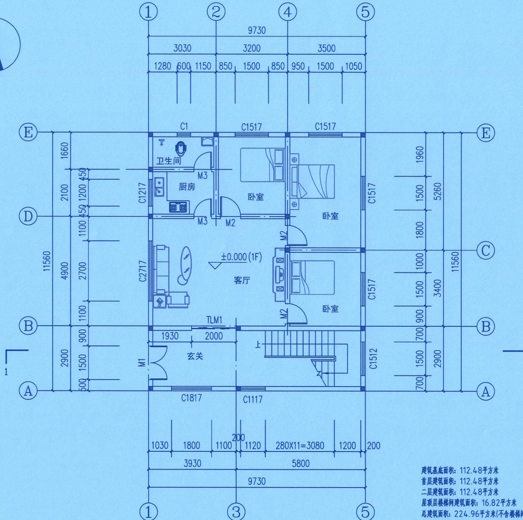
首层平面图 1:100
