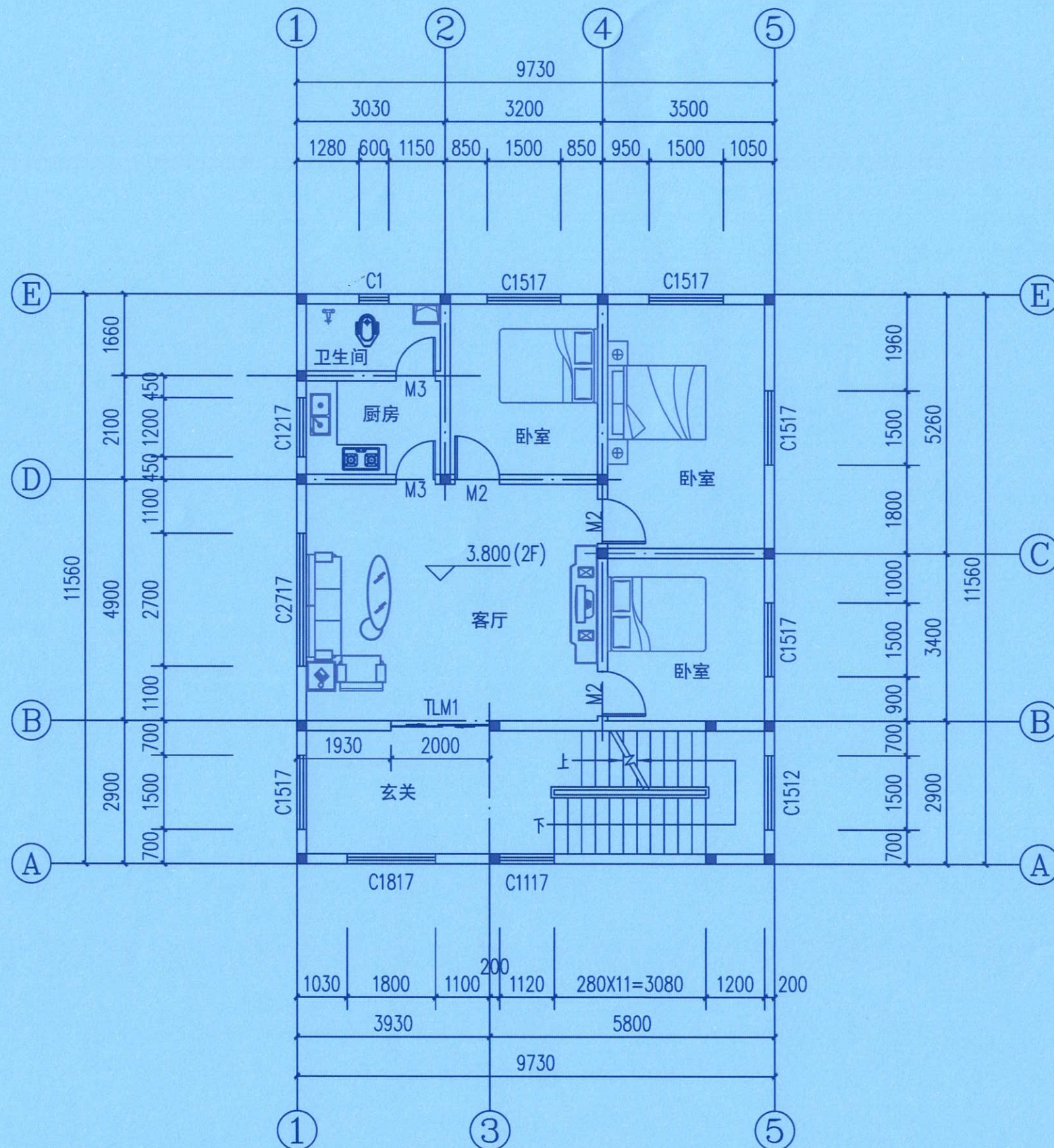
二层平面图 1:100
