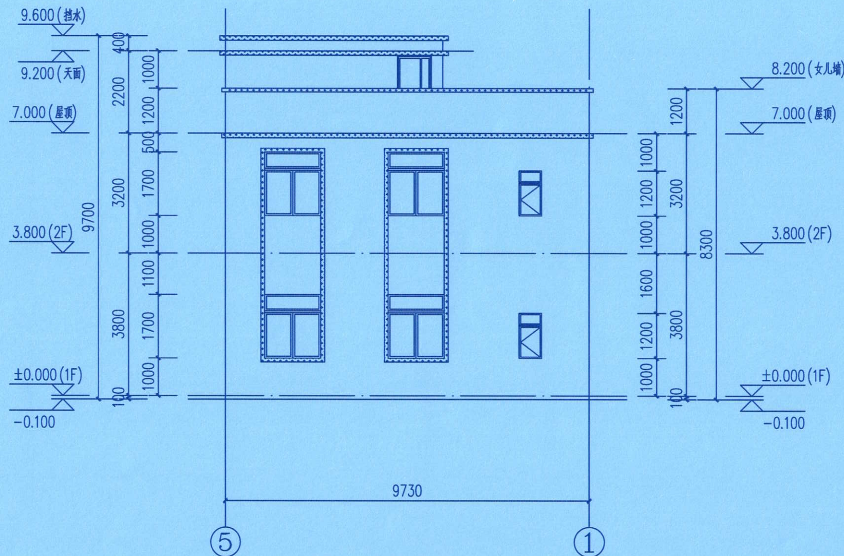
⑤-①轴立面图 1:100
