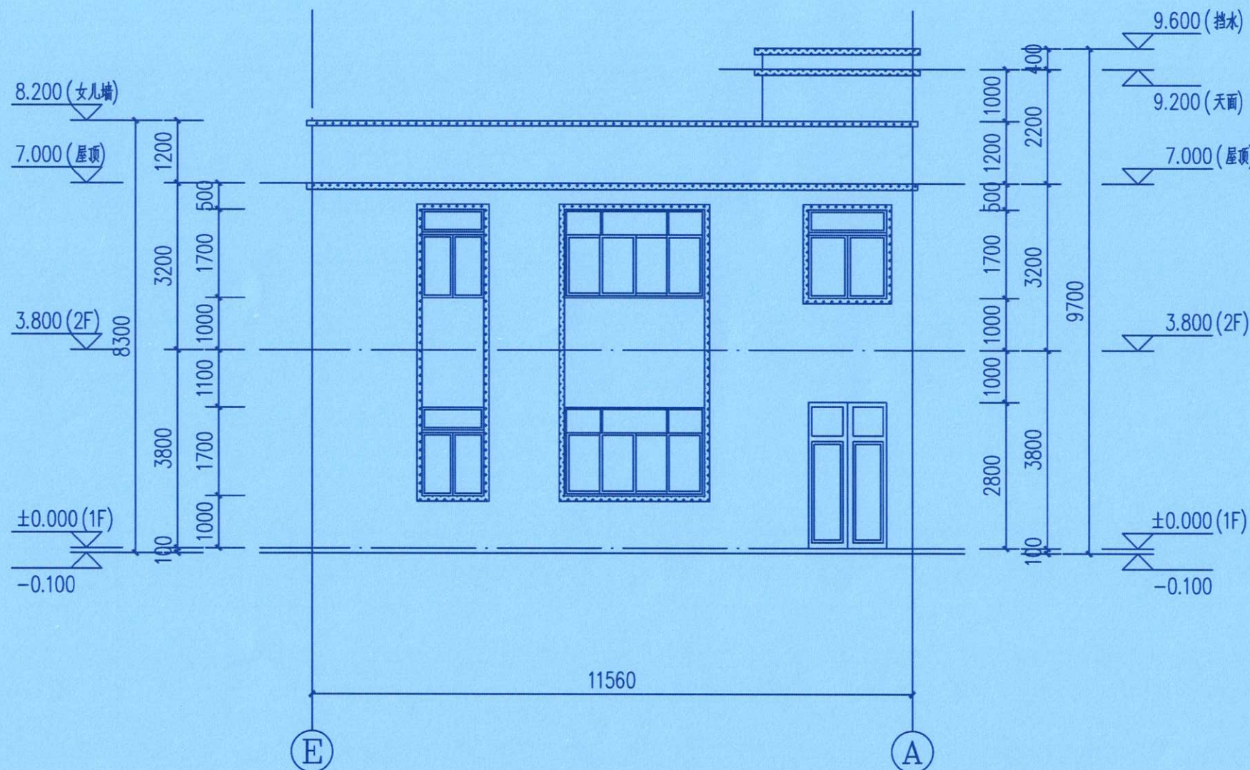
①-②轴立面图 1:100
