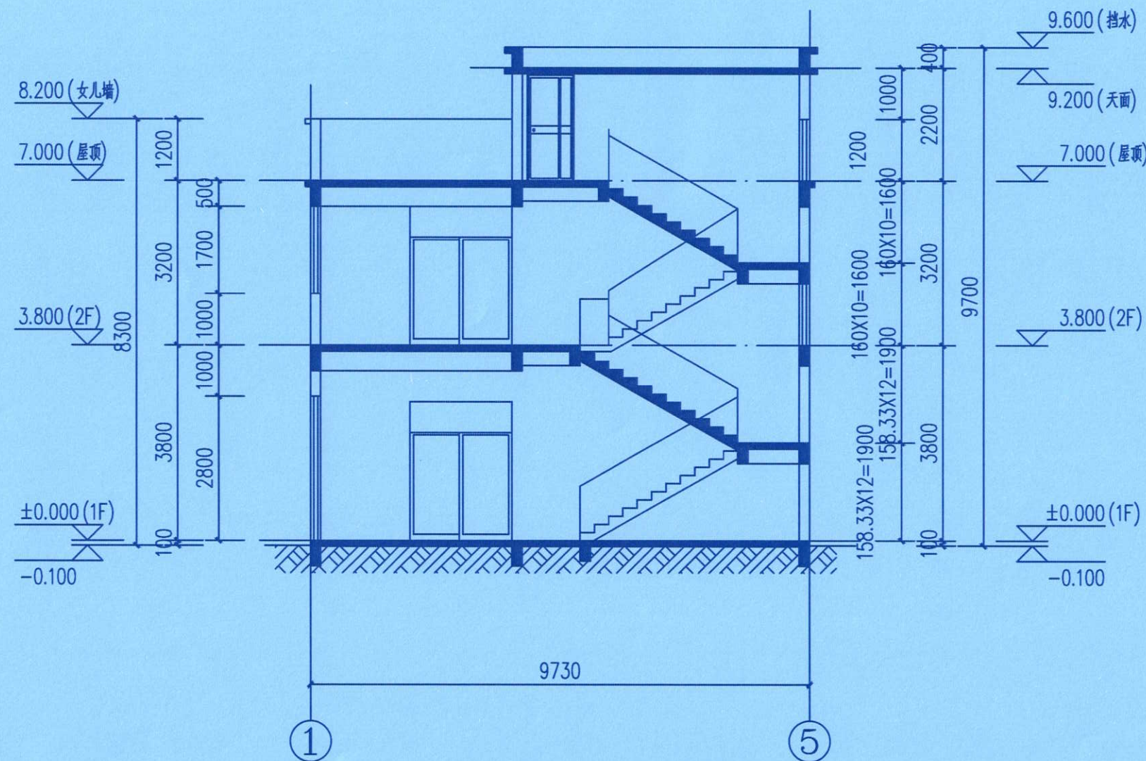
1-1剖面图 1:100
