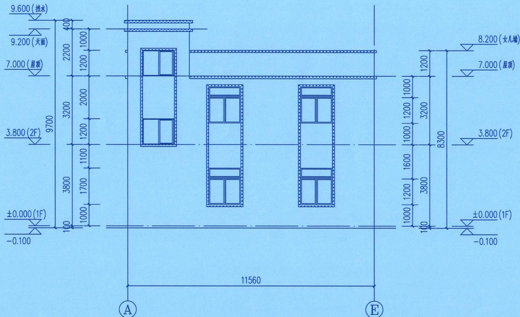
①-⑤轴立面图 1:100
