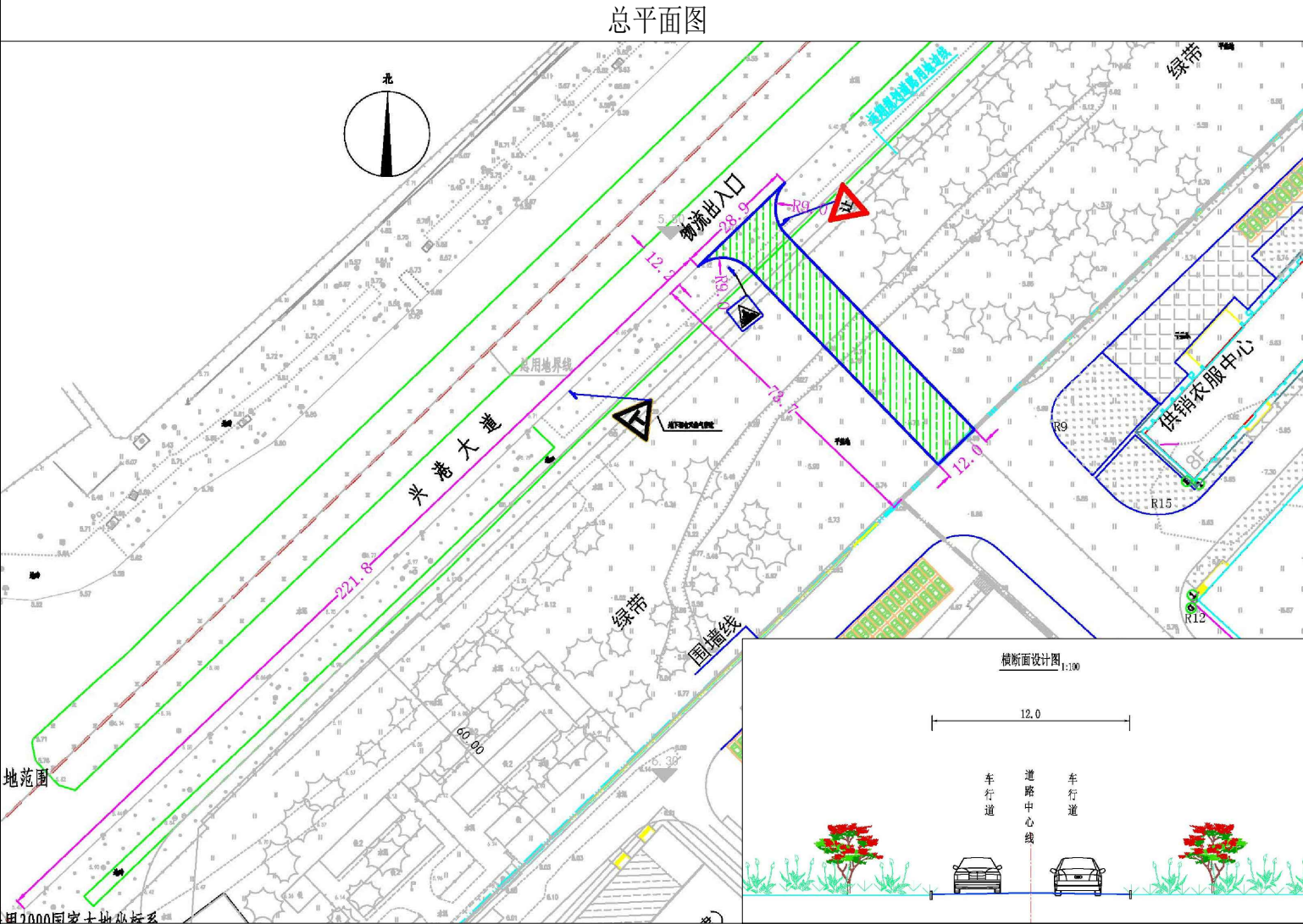
兴港大道开设一个28.9米—12米宽，长73.7米路口(双向), 其中标准横断面设计图为12米双向机动车道。
