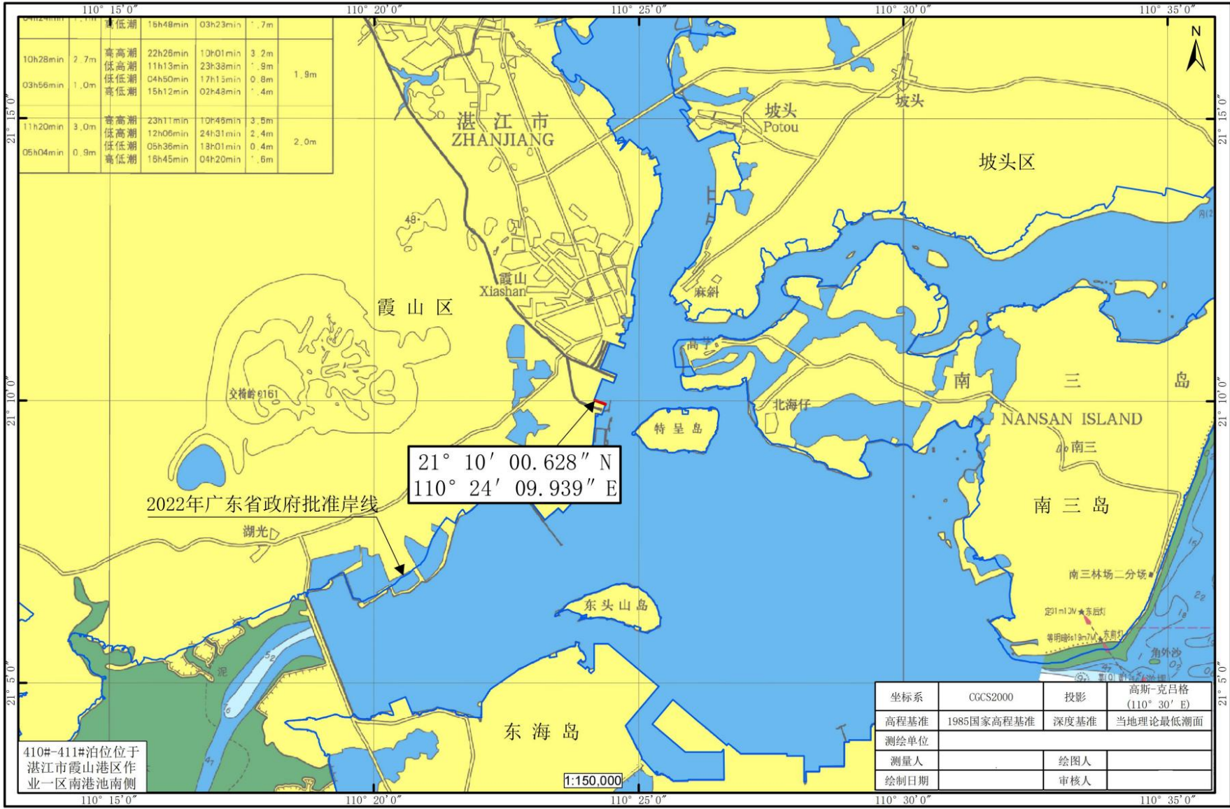
湛江港霞山港区410#-411#泊位升级改造工程宗海位置图
